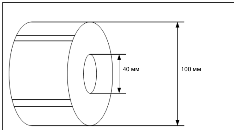
Рисунок 1.8 – Геометрические размеры рулона
