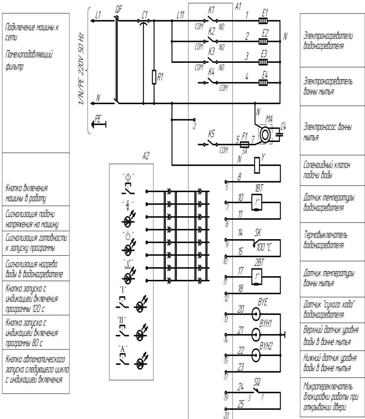
Рисунок 3 (лист 1 из 2)– Схема электрическая принципиальная
