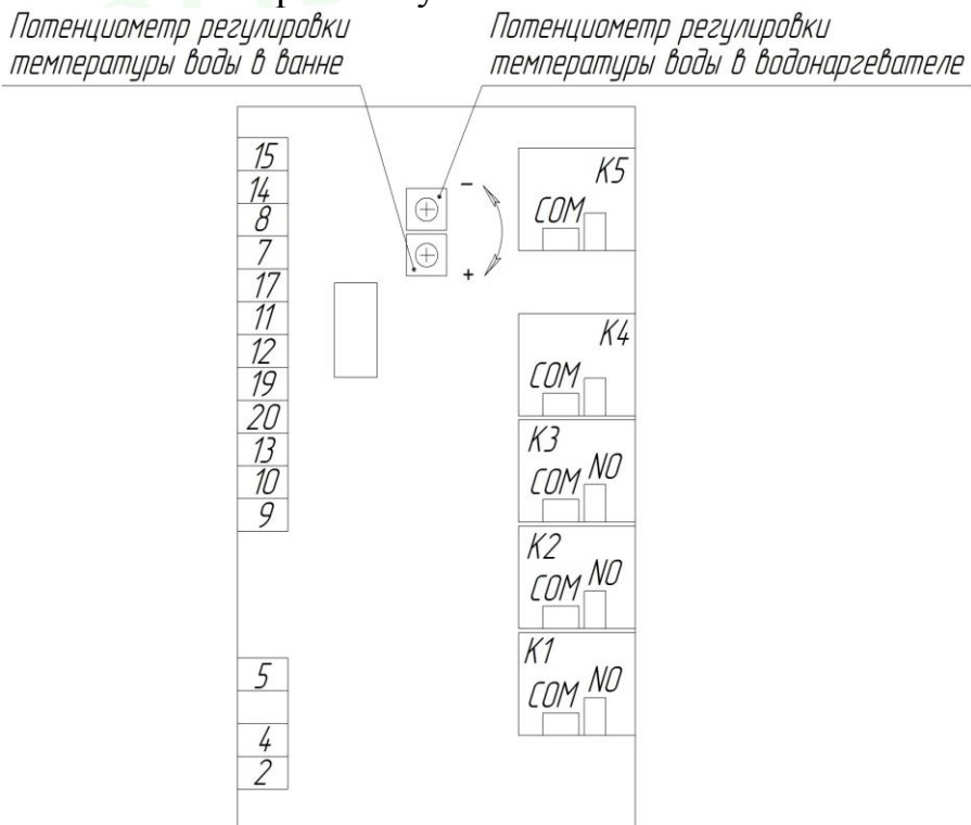
Рисунок 2 – Условное обозначение контактов блока управления
