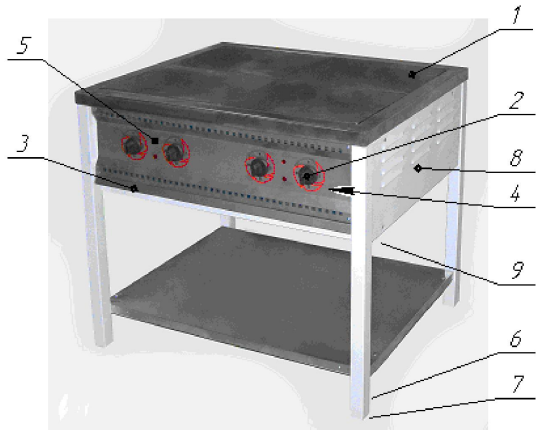
Рисунок 1. Загальний вигляд плити: 1 - конфорка; 2 — перемикач потужності конфорки; 3 - піддон-жирозбірник; 4 - панель управління; 5 - лампа сигнальна; 6 - захисний затискач (заземлення); 7 - опора регулююча; 8 - клемна коробка для вводу кабеля.
