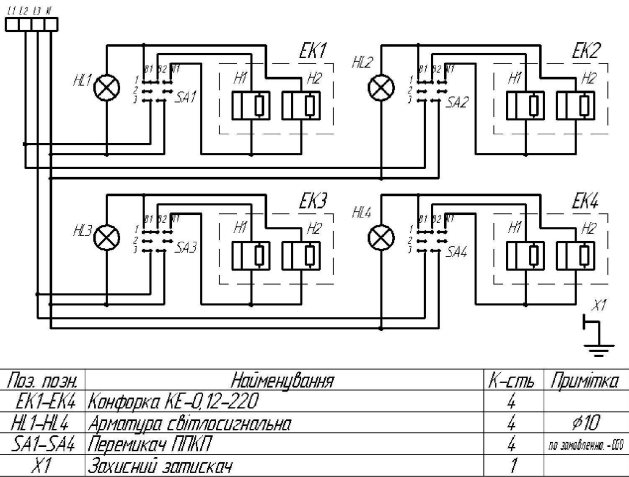
Рисунок 2. Схема електрична принципова
